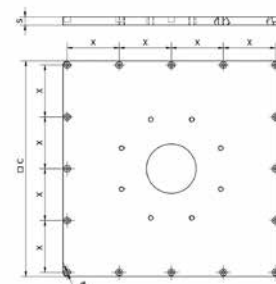
Nr16 Chemische Dübel GEGENPLATTE Z2
