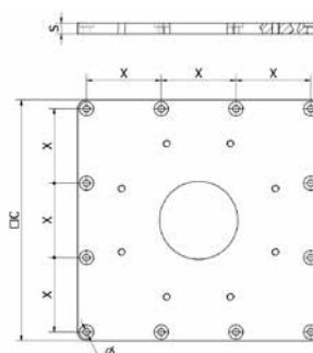
Nr12 Chemische Dübel GEGENPLATTE U - V - Z1
