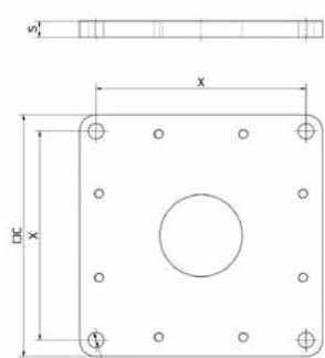
Nr4 Chemische Dübel GEGENPLATTE R - S
